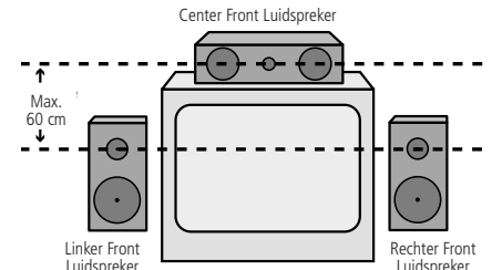
A) Installatie Front Luidsprekers met Gewone TV of Achter Projectie TV
